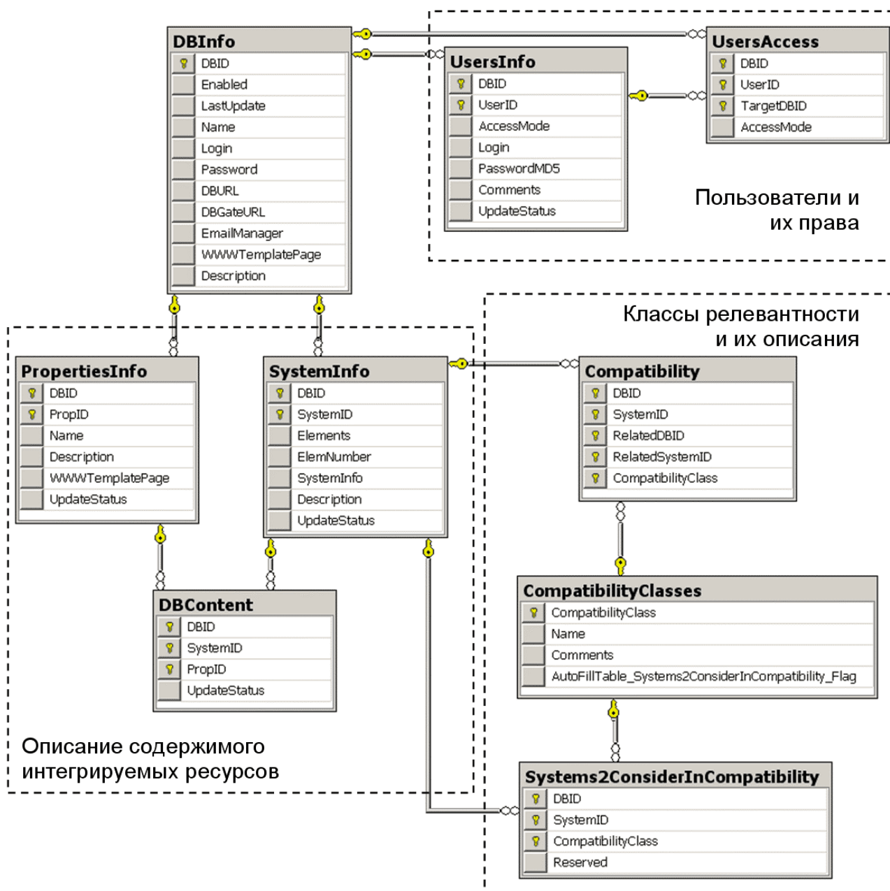
Рис. 7. Структура метабазы для интеграции Web-приложений ИС.
