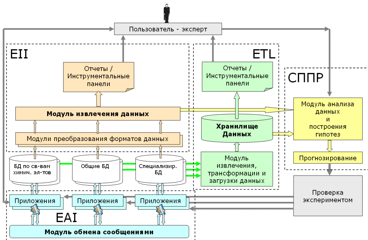
Рис. 3. Анализ информационных потоков при использовании разных подходов к интеграции и место интегрированной ИС в СППР.
