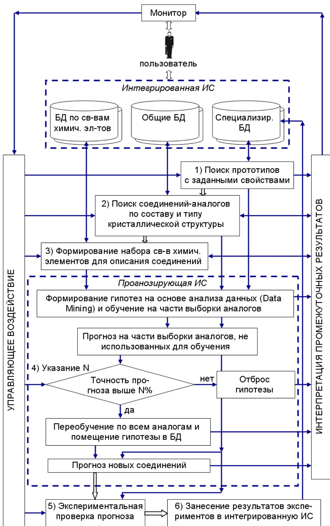
Рис. 9. Методика использования интегрированной ИС в СПДР.
