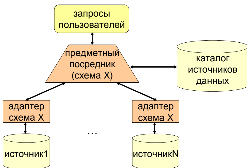
Рис. 4. Интеграция на основе принципа Local-As-View.
