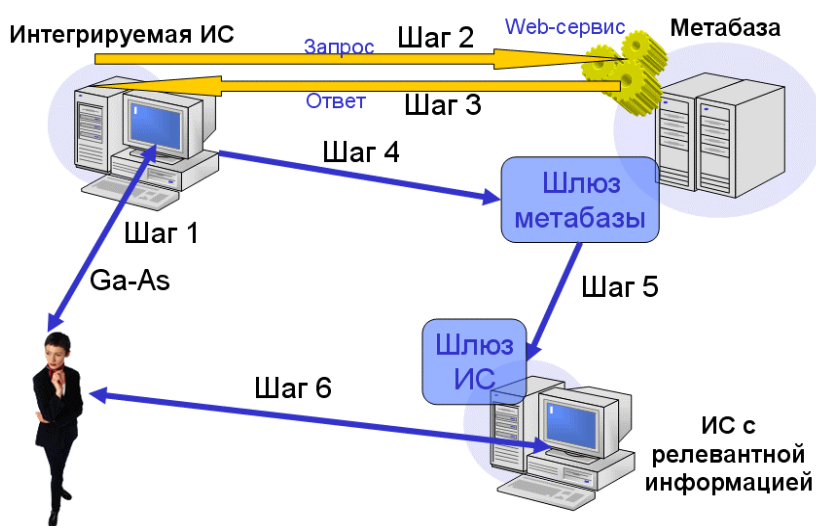
Рис. 5. Интеграция Web-приложений ИС с поиском релевантной информации в метабазе.
